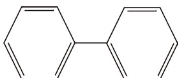
Bifenilo
