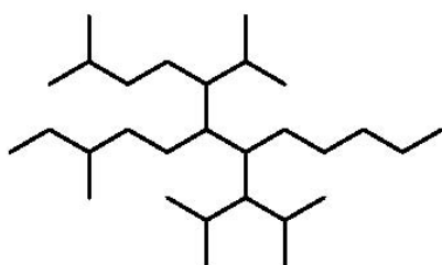
2-metil-5-(1-metiletil)-7-(2-metil-1-(1-metiletil)propil)- 6-(3-metilpentil)dodecano
