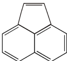
Acenafaileno
