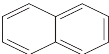
Naftaleno
